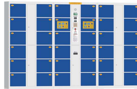
BS-EL-36 H1800*W2550*D460mm
