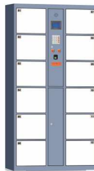
BS-EL-12 H1800*W850*D460mm
