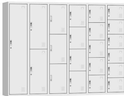
BS-SL-01/02/03/04/05/06 H1850*W380*D420mm
